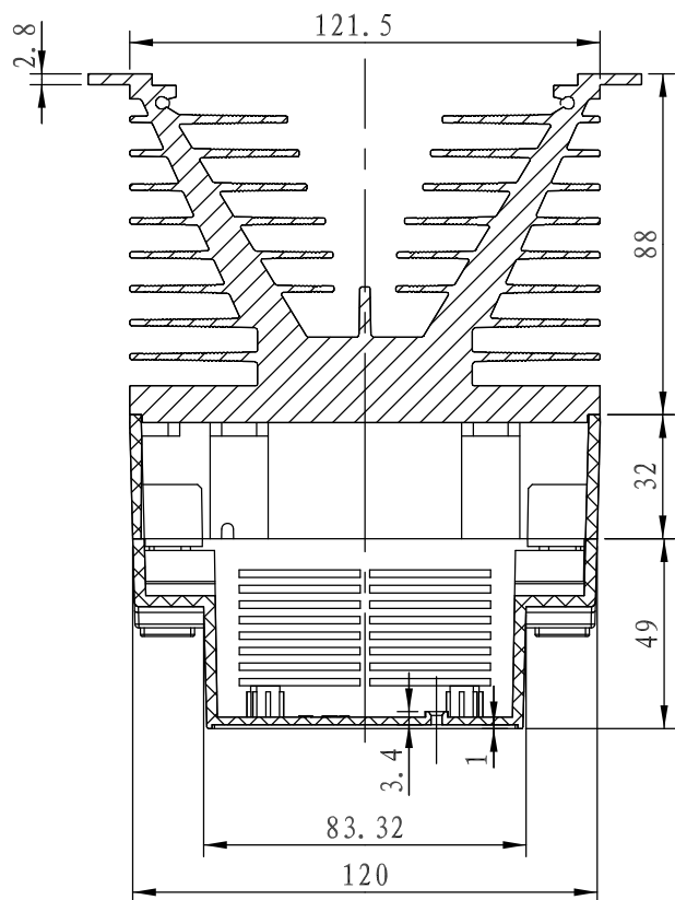
剖面 A-A
