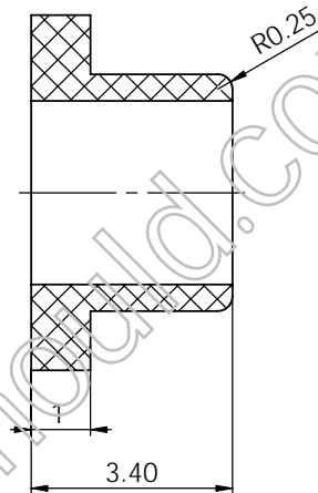
剖面 A-A
